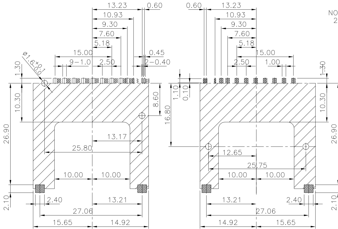
RECOMMEND PCB LAYOUT : \pm 0.05\text{mm} (Reverse type)
